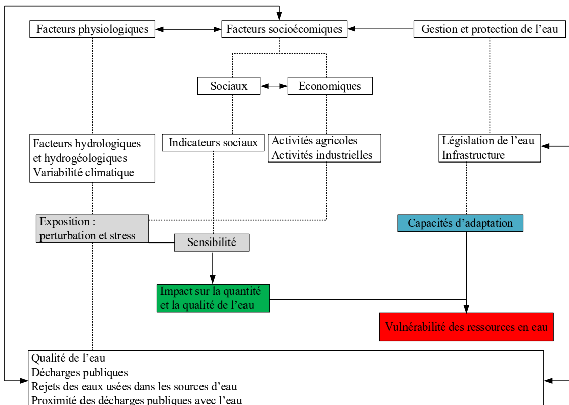
Figure 1: Exemple d'un cadre conceptuel de l'évaluation de la vulnérabilité des ressources en eau
